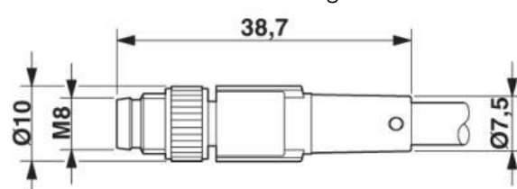
Stecker M8 x 1, gerade
