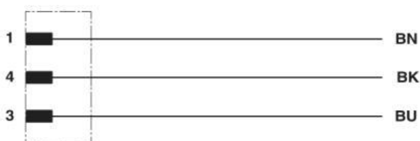
Kontaktbelegung des M8-Steckers
