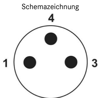
Polbild M8-Stecker, 3-polig, A-kodiert, Ansicht Stiftseite
