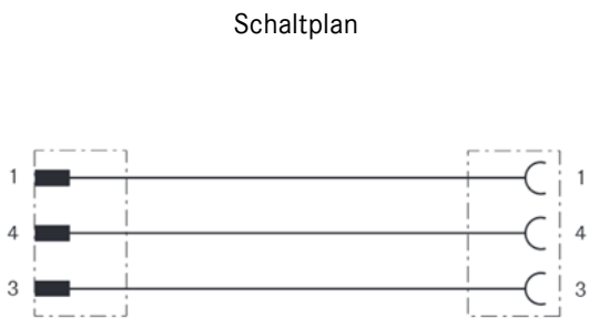
Kontaktbelegung des M8-Stecker und der M12-Buchse
