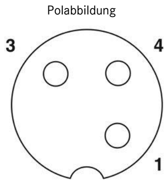
Polbild M12-Buchse, 3-polig, A-kodiert, Ansicht Buchsenseite
