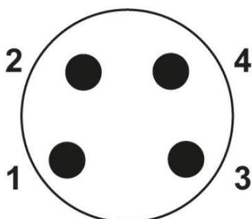
Polbild M8-Stecker, 4-polig, A-kodiert, Ansicht Stiftseite
