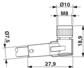
Maßzeichnung
