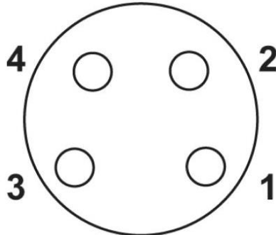
Pin assignment M8-jack, 4-pol, A-codiert
