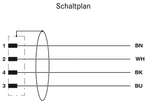
Kontaktbelegung des M12-Steckers
