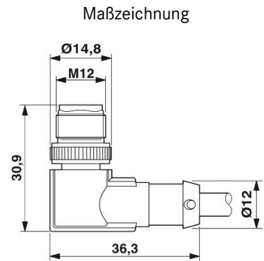
Stecker M12 x 1, gewinkelt, geschirmt
