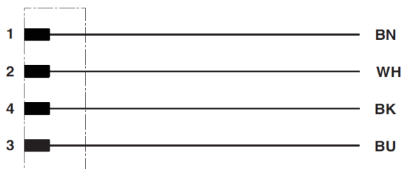
Kontaktbelegung des M12-Steckers
