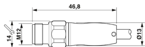
Maßzeichnung
