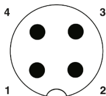
Polbild M12-Stecker, 4-polig, A-kodiert, Ansicht Stiftseite
