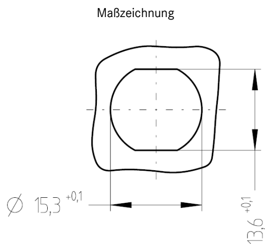
Blechausschnitt für Verdrehschutz
