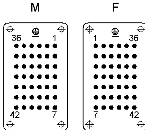
Polbild, Kabelanschlusseite
