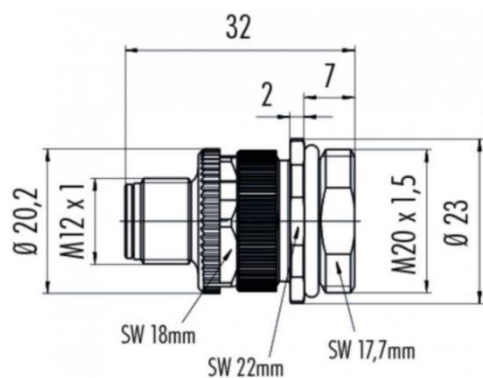
Flanschstecker
