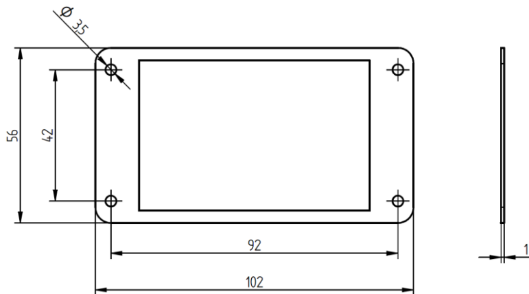
Flachdichtung, H-A 32 (10607600)
