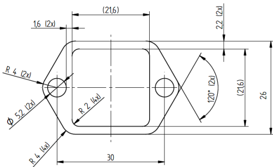
Flachdichtung, H-A 3 (38116823)
