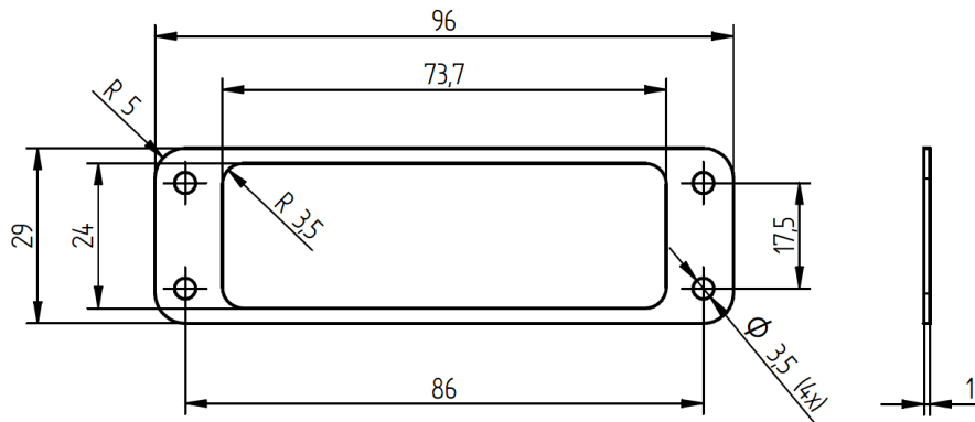
Flachdichtung, H-A 16 (10607300)
