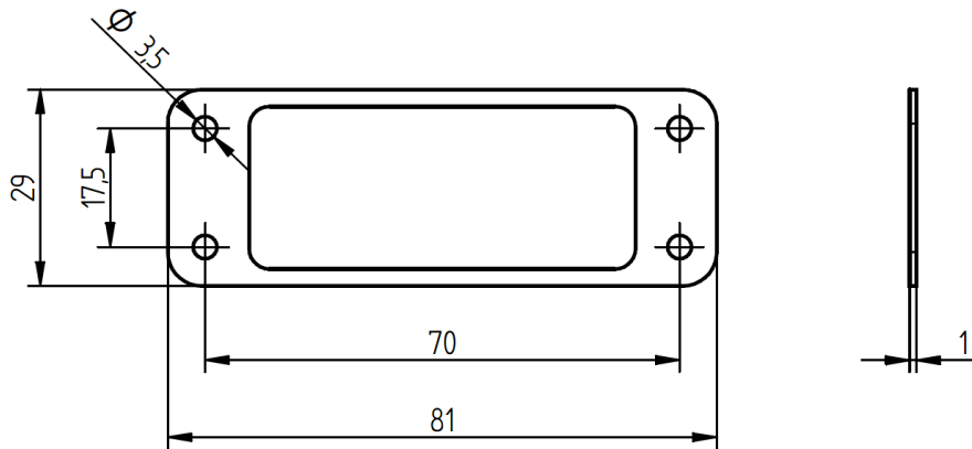
Flachdichtung, H-A 10 (10607200)
