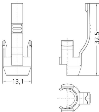
Maßzeichnung
