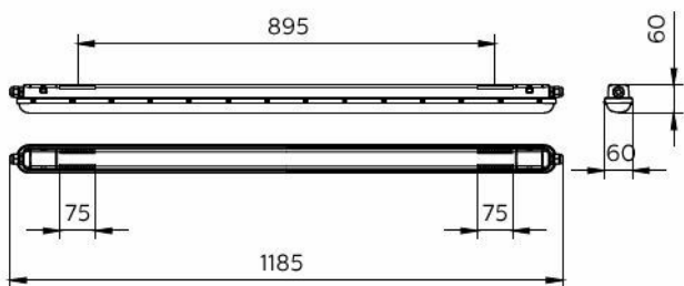
WT008C L1200 TW
