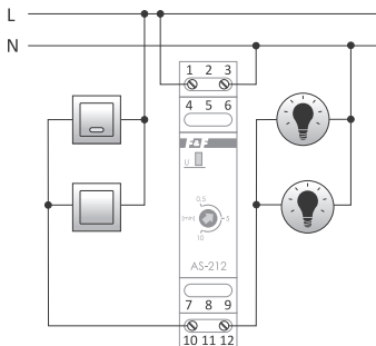
câblage à 4 fils
