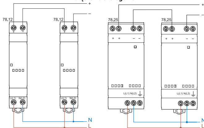
Połączenia szeregowe
