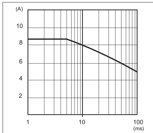
P78-6 Szczytowy prąd wyjścia w czasie (78.50)
