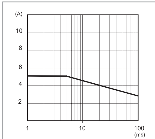
P78-5 Szczytowy prąd wyjścia w czasie (78.60)
