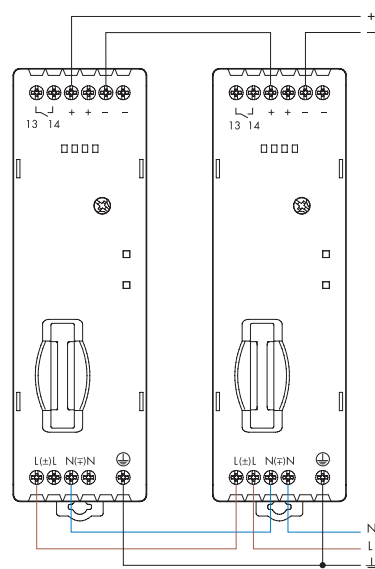
Połączenia szeregowe
