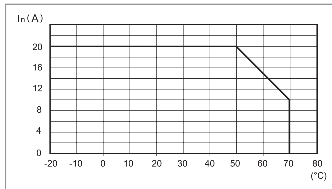
L78-15 Wykres poziomu prądu wyjściowego względem temperatury otoczenia (78.Y1)
