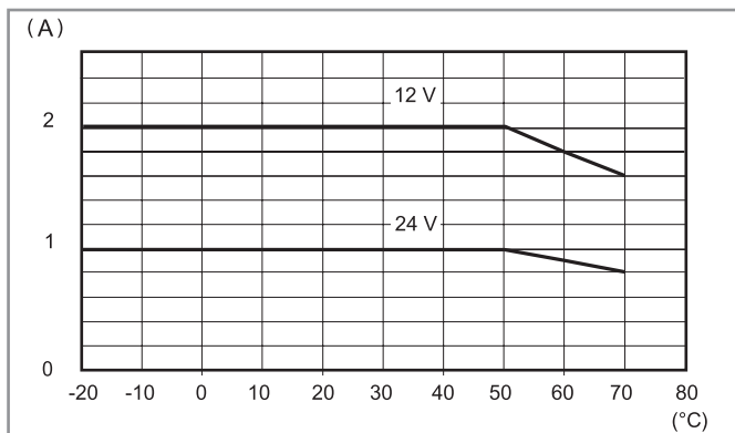
L78-3 Wykres poziomu prądu wyjściowego względem temperatury otoczenia (78.25)
