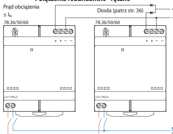
Połączenia redundantne - ręczne
