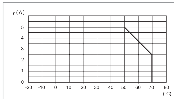
L78-13 Wykres poziomu prądu wyjściowego względem temperatury otoczenia (78.W1)
