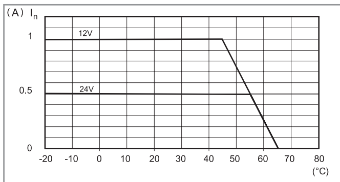
L78-2 Wykres poziomu prądu wyjściowego względem temperatury otoczenia (78.12-1202/2402)
