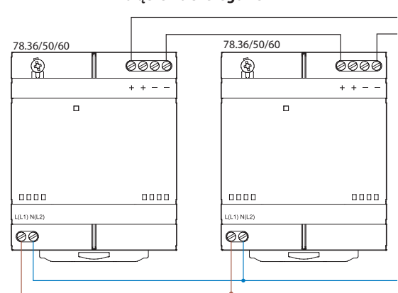
Połączenia szeregowe
