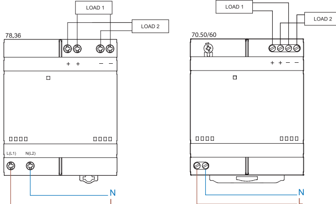
Połączenie dualne
