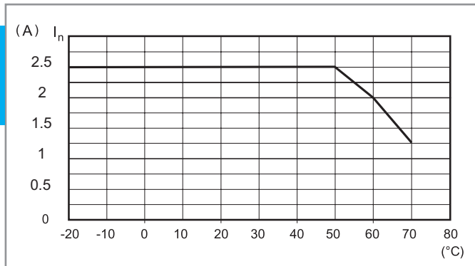
L78-5 Wykres poziomu prądu wyjściowego względem temperatury otoczenia (78.60)
