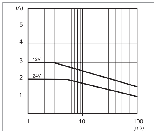
P78-2 Szczytowy prąd wyjścia w czasie (78.12-xxxx)
