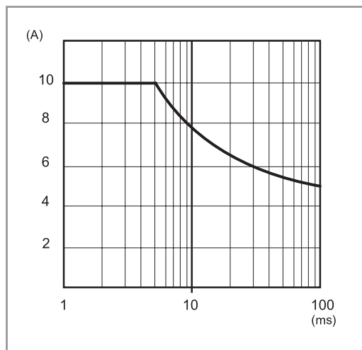
P78-9 Szczytowy prąd wyjścia w czasie (78.1D)
