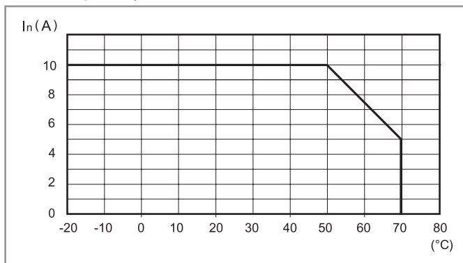
L78-14 Wykres poziomu prądu wyjściowego względem temperatury otoczenia (78.X1)
