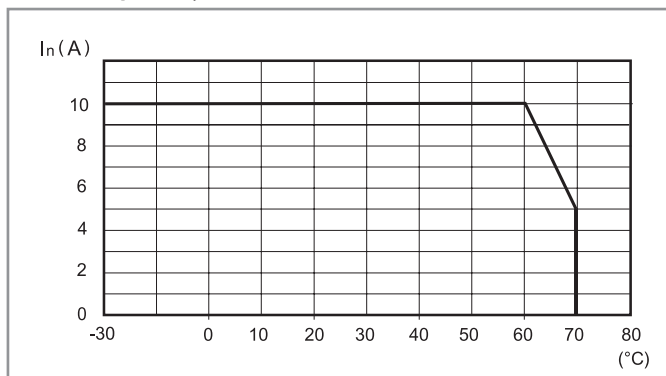
L78-20 Wykres poziomu prądu wyjściowego względem temperatury otoczenia (78.X3)
