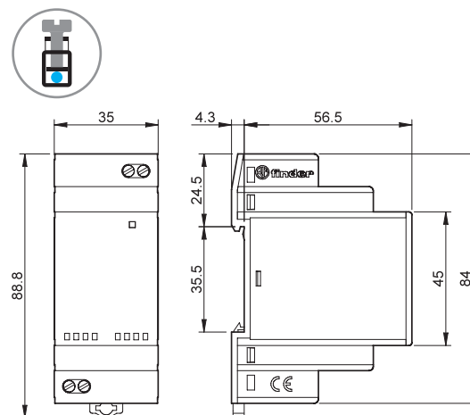
Typ 78.25-2482 Zaciski śrubowe (koszyczkowe)
