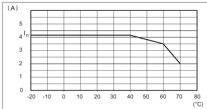
L78-6 Wykres poziomu prądu wyjściowego względem temperatury otoczenia (78.50)
