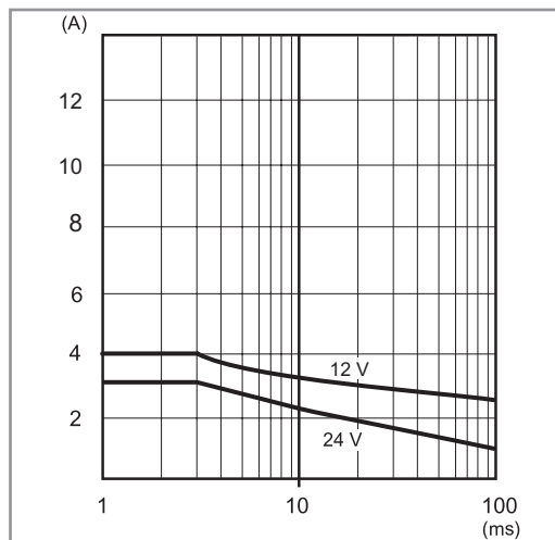
P78-3 Szczytowy prąd wyjścia w czasie (78.25)
