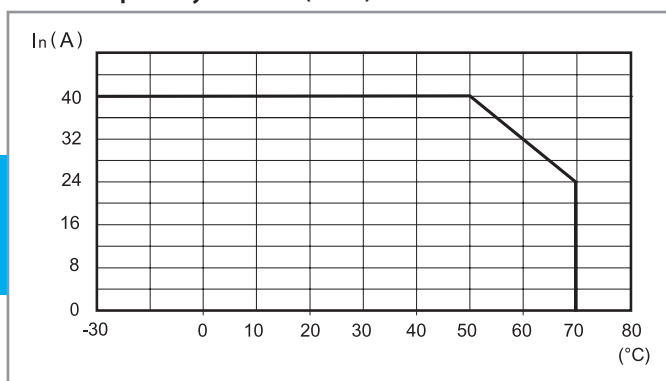
L78-22 Wykres poziomu prądu wyjściowego względem temperatury otoczenia (78.Z3)
