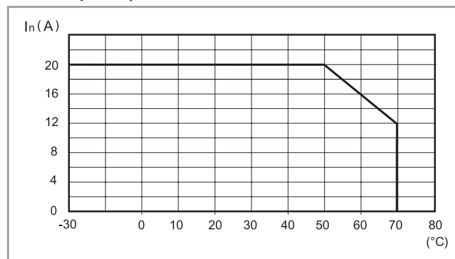
L78-19 Wykres poziomu prądu wyjściowego względem temperatury otoczenia (78.Y2)
