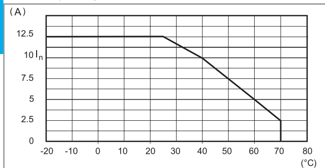
L78-11 Wykres poziomu prądu wyjściowego względem temperatury otoczenia (78.2E)
