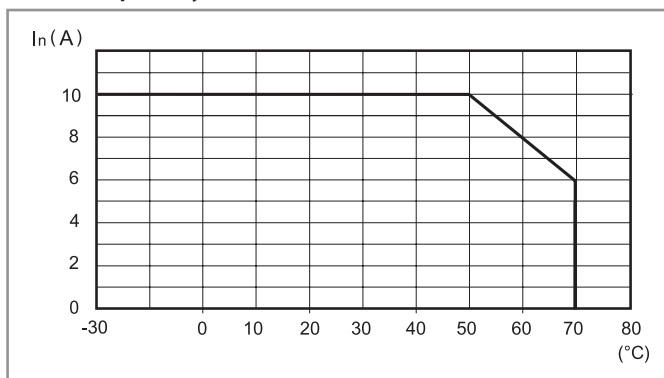
L78-18 Wykres poziomu prądu wyjściowego względem temperatury otoczenia (78.X2)
