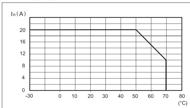
L78-21 Wykres poziomu prądu wyjściowego względem temperatury otoczenia (78.Y3)
