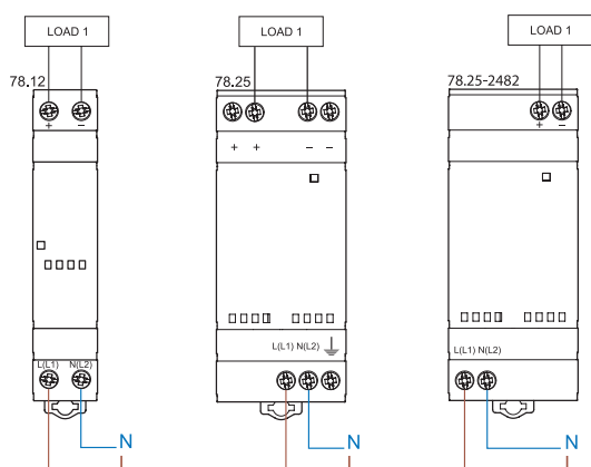
Połączenie dualne
