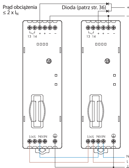
Połączenia równoległe
