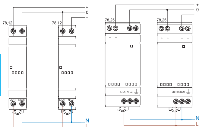
Połączenia szeregowe
