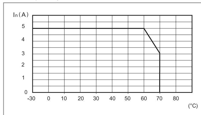
L78-17 Wykres poziomu prądu wyjściowego względem temperatury otoczenia (78.W2)
