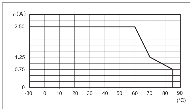
L78-16 Wykres poziomu prądu wyjściowego względem temperatury otoczenia (78.H2)
