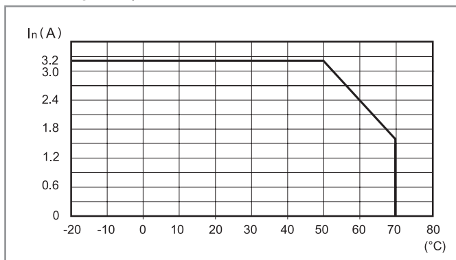
L78-12 Wykres poziomu prądu wyjściowego względem temperatury otoczenia (78.J1)
