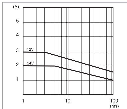
P78-3 Szczytowy prąd wyjścia w czasie (78.25)
