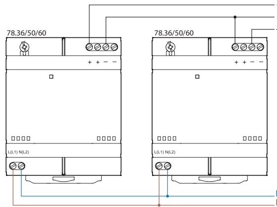
Połączenia szeregowe
