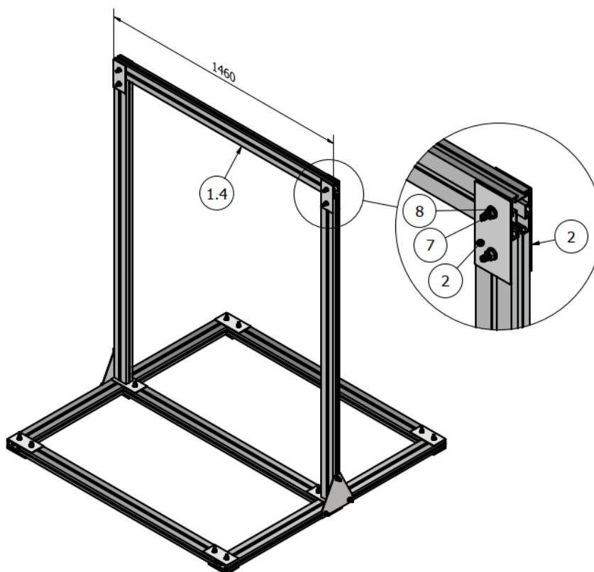
RYŚ. 5 Montaż belki poziomej górnej
