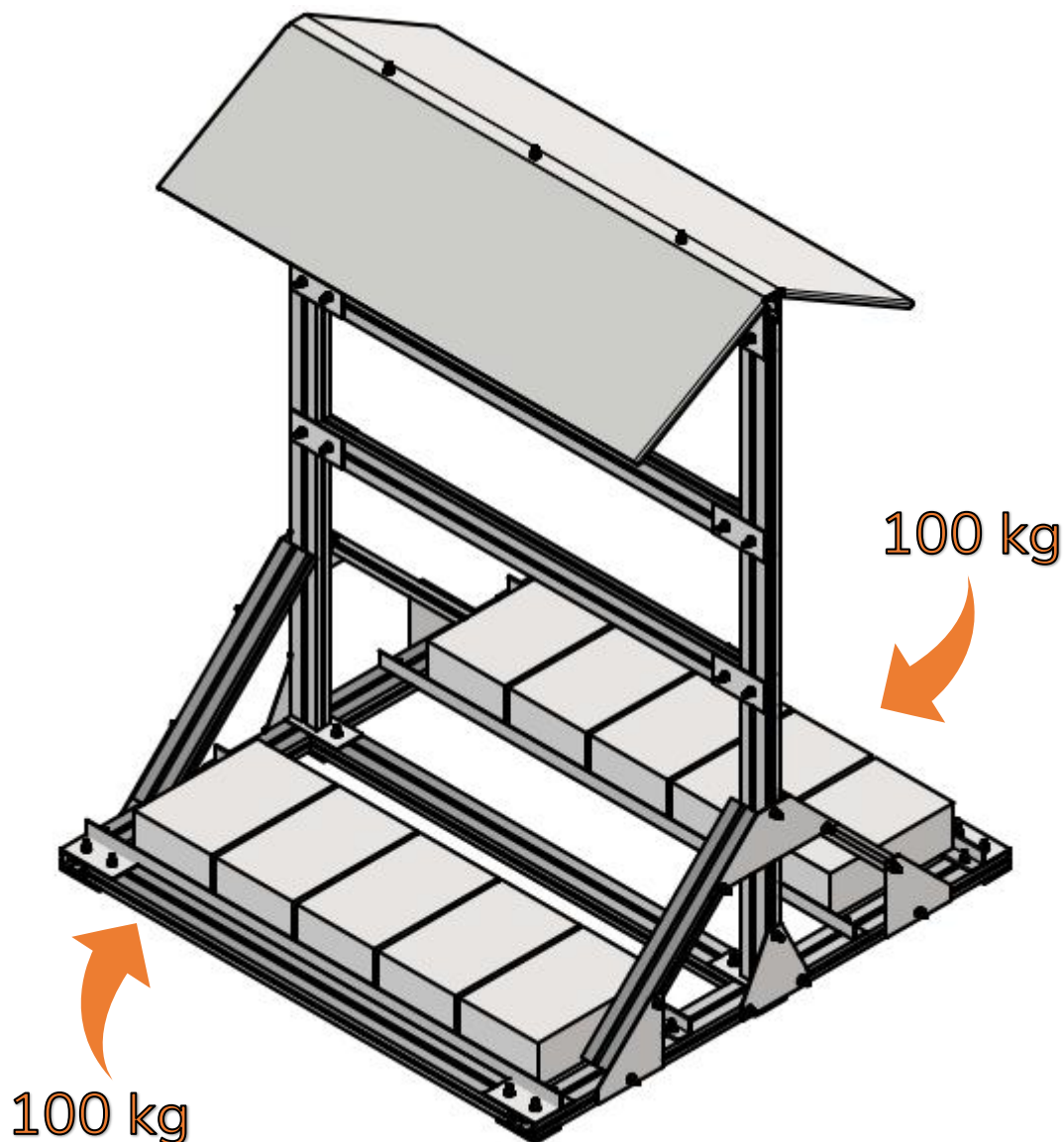
RYS. 12 Ułożenie balastu
