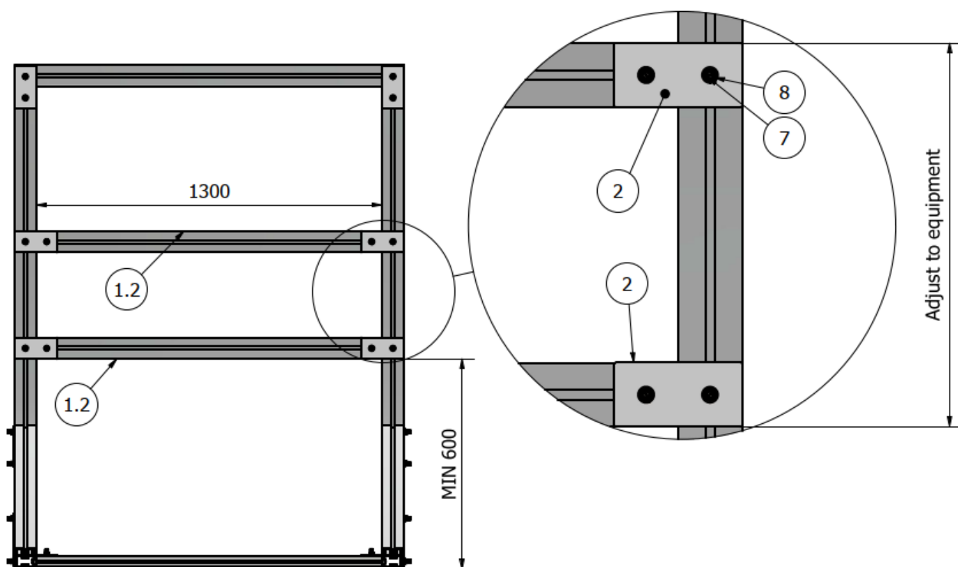
RYS. 9 Montaż poprzeczek v1.1
