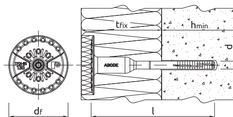
Montaż zagłębiony
