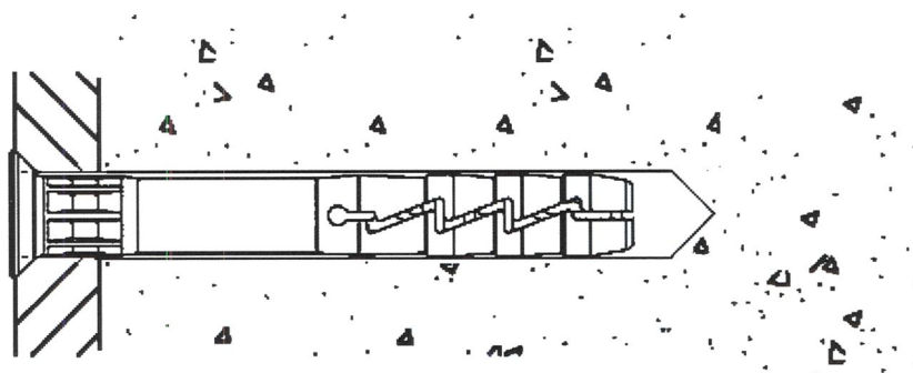
Rysunek A5. Mocowanie z zastosowaniem tworzywowo-metalowego łącznika rozporowego FX w wariancie L
