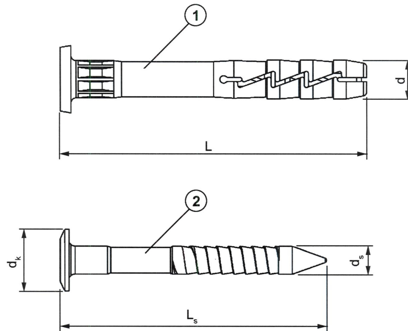
Rysunek A3. Elementy składowe tworzywowo-metalowych łączników rozporowych FX w wariantcie C, w wersjach 05, 06 i 08, z tuleją tworzywową z polipropylenu lub poliamidu 1 – tuleja tworzywowa, 2 – trzpień stalowy
