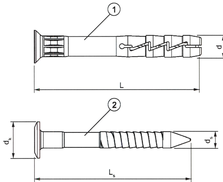
Rysunek A1. Elementy składowe tworzywowo-metalowych łączników rozporowych FX w wariantcie L, w wersjach 05, 06 i 08, z tuleją tworzywową z polipropylenu lub poliamidu 1 – tuleja tworzywowa, 2 – trzpień stalowy
