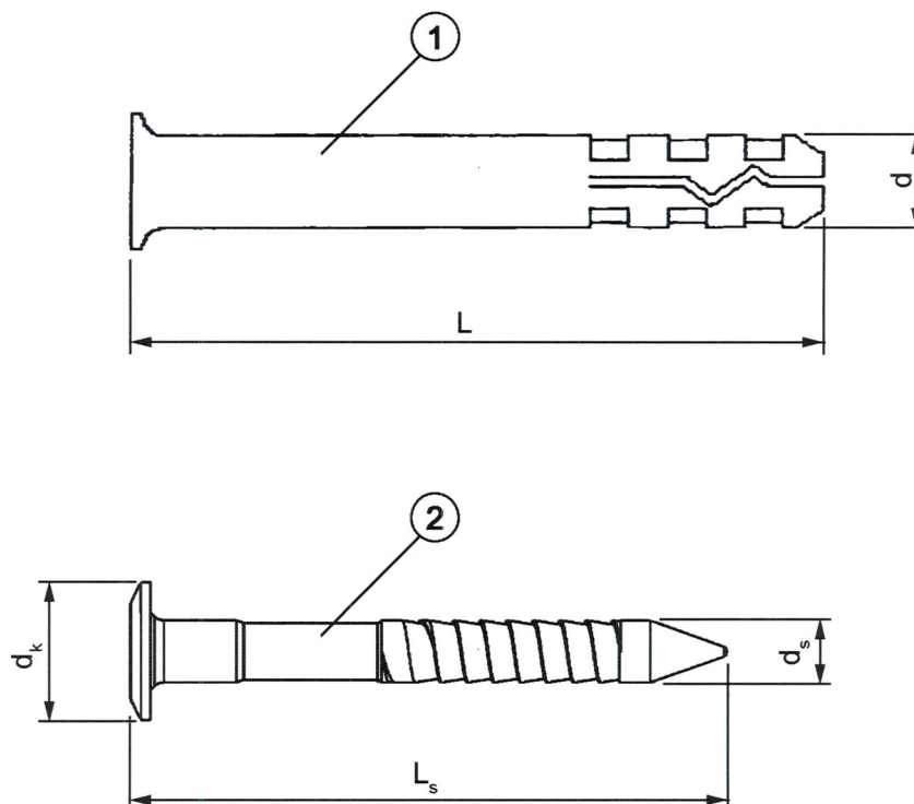
Rysunek A4. Elementy składowe tworzywowo-metalowych łączników rozporowych FX w wariantcie L, w wersji 10, z tuleją tworzywową z poliamidu 1 – tuleja tworzywowa, 2 – trzpień stalowy
