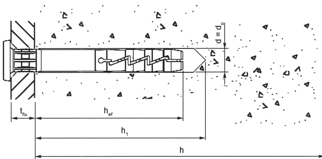
Rysunek B2. Parametry montażu tworzywowo-metalowych łączników rozporowych FX w wariantie C
