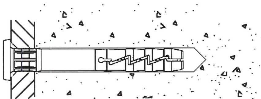
Rysunek A6. Mocowanie z zastosowaniem tworzywowo-metalowego łącznika rozporowego FX w wariancie C
