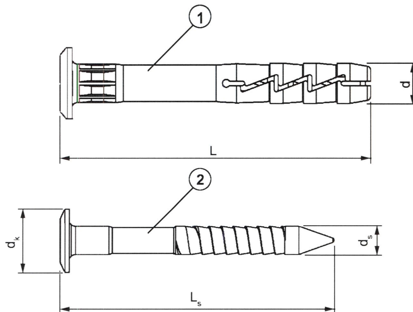
Rysunek A2. Elementy składowe tworzywowo-metalowych łączników rozporowych FX w wariantcie K, w wersjach 05, 06 i 08, z tuleją tworzywową z polipropylenu lub poliamidu 1 – tuleja tworzywowa, 2 – trzpień stalowy
