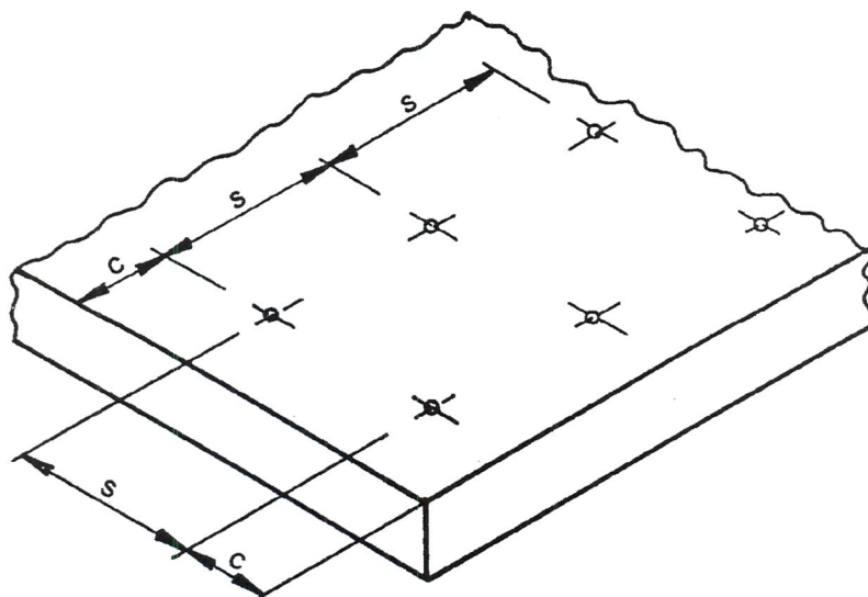
Rysunek B3. Parametry rozmieszczenia tworzywowo-metalowych łączników rozporowych FX w podłożu s – rozstaw osiowy łączników, c – odległość łącznika od krawędzi podłoża
