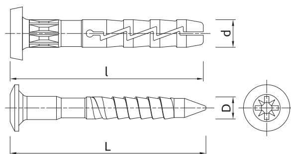
Wymiary produktu
