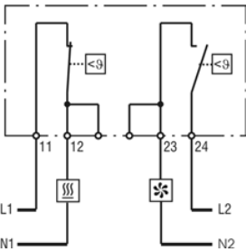
Schemat połączeń Termostat ZR 011
