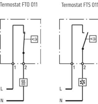
Schemat połączeń
