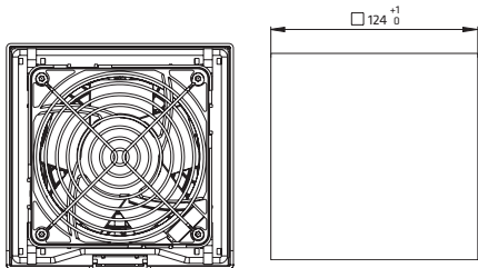
WYKRÓJ MONTAŻOWY
