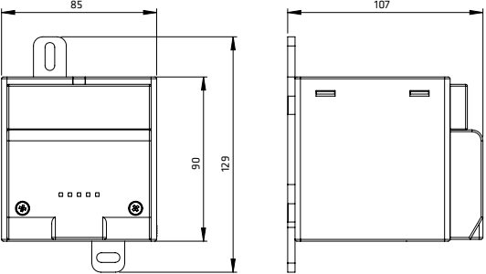
Dmuchawa grzewcza CSL 028
