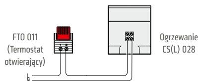
Przykład podłączenia
