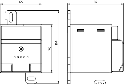
Dmuchawa grzewcza CS 028
