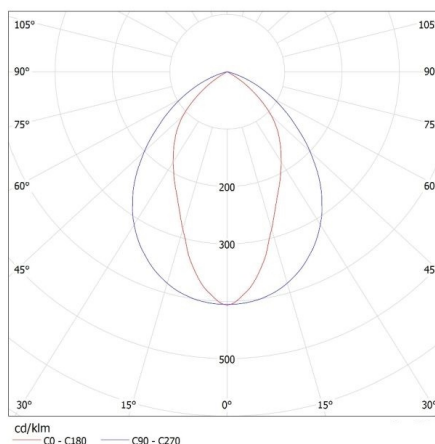
KANLUX S.A. (kat 19733) NOTUS 3 EVG 218 NT / Krzywa rozsyłu światła (biegunowo)
