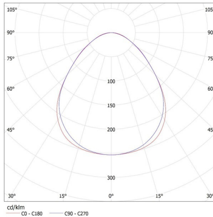
KANLUX S.A. (kat 28442) AL 4LED 60-MPR-SR-NT + GLASSv4 / LDC (Polar)
