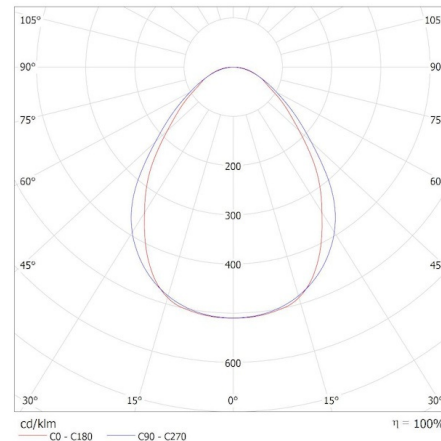
KANLUX S.A. (kat 35615) AL-MS-WW-MPR-W-PT / Krzywa rozsyłu światła (biegunowo)
