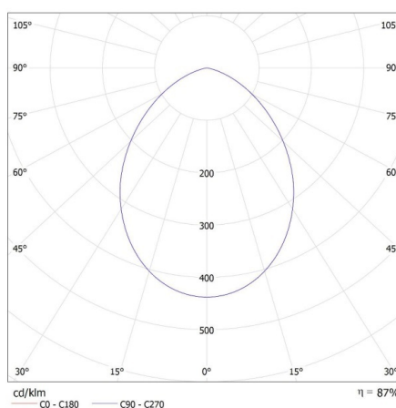
KANLUX S.A. (kat 35670) TIBERI PRO 20W-940-W / LDC (Polar)
