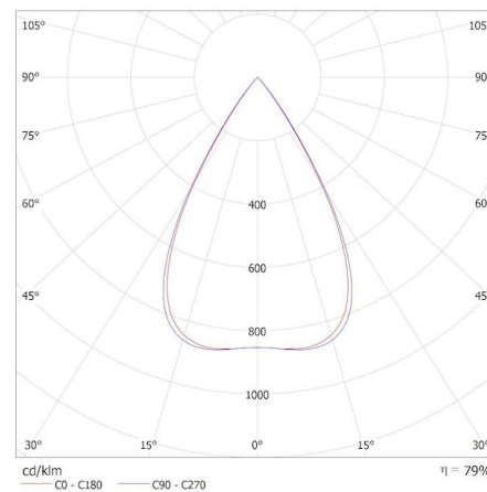
KANLUX S.A. (kat 35942) OS-L5D-WW-RST-B-N1 / Krzywa rozsyłu światła (biegunowo)
