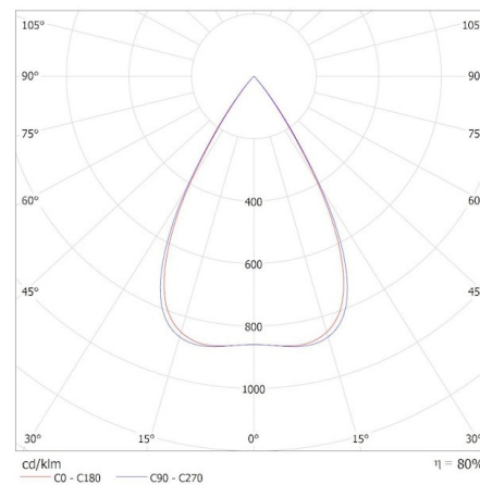
KANLUX S.A. (kat 35954) OS-S5D-NW-RST-B-N1 / Krzywa rozsyłu światła (biegunowo)
