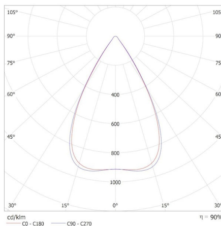
KANLUX S.A. (kat 36071) OS-L5D-WN-RST-W-N3 / Krzywa rozsyłu światła (biegunowo)
