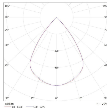
KANLUX S.A. (kat 36151) OS-L8D-WN-RST-B-N3 / Krzywa rozsyłu światła (biegunowo)
