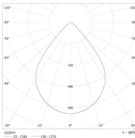
KANLUX S.A. (kat 37180) OS-S8D-WW-RX-W-P1 / Krzywa rozsyłu światła (biegunowo)
