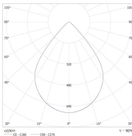
KANLUX S.A. (kat 37181) OS-L8D-WW-RX-W-P1 / Krzywa rozsyłu światła (biegunowo)
