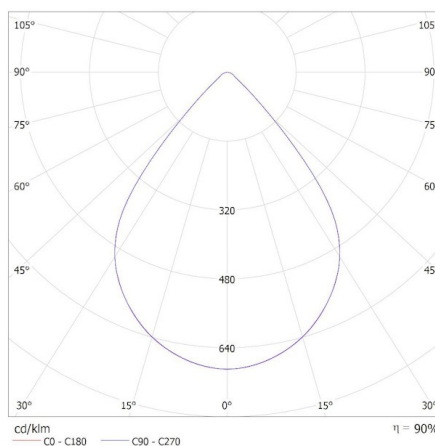
KANLUX S.A. (kat 37185) OS-L8D-WN-RX-W-P1 / Krzywa rozsyłu światła (biegunowo)
