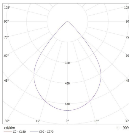
KANLUX S.A. (kat 37186) OS-M8D-WN-RX-W-P1 / Krzywa rozsyłu światła (biegunowo)
