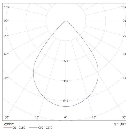
KANLUX S.A. (kat 37189) OS-L8D-NW-RX-W-P1 / Krzywa rozsyłu światła (biegunowo)
