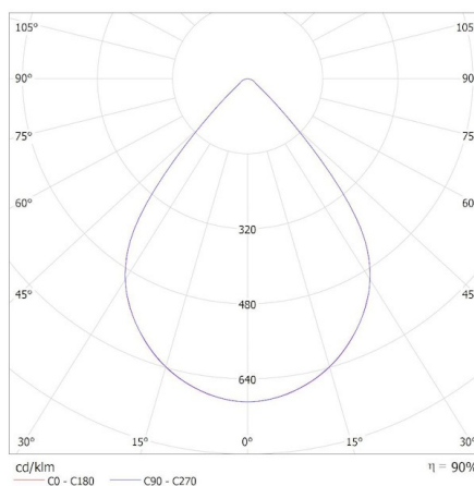
KANLUX S.A. (kat 37190) OS-M8D-NW-RX-W-P1 / Krzywa rozsyłu światła (biegunowo)
