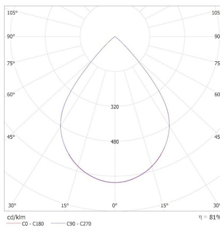
KANLUX S.A. (kat 37192) OS-S8D-WW-RX-B-P1 / Krzywa rozsyłu światła (biegunowo)
