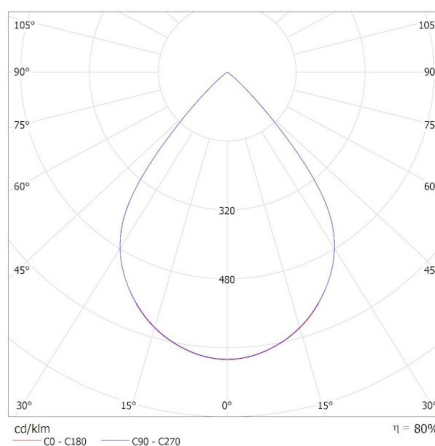
KANLUX S.A. (kat 37193) OS-L8D-WW-RX-B-P1 / Krzywa rozsyłu światła (biegunowo)
