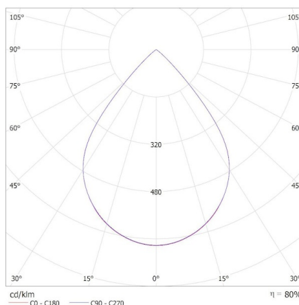
KANLUX S.A. (kat 37194) OS-M8D-WW-RX-B-P1 / Krzywa rozsyłu światła (biegunowo)
