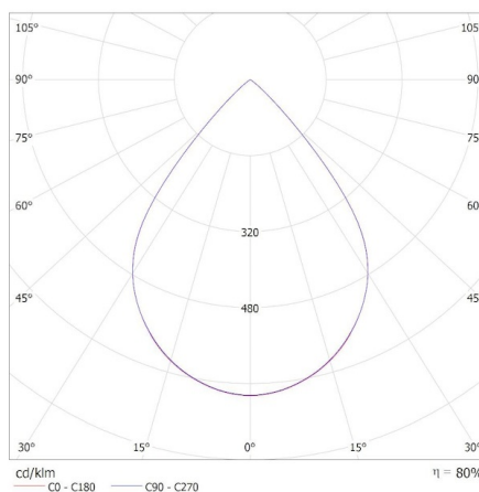
KANLUX S.A. (kat 37196) OS-S8D-WN-RX-B-P1 / Krzywa rozsyłu światła (biegunowo)
