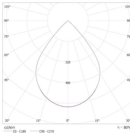
KANLUX S.A. (kat 37197) OS-L8D-WN-RX-B-P1 / Krzywa rozsyłu światła (biegunowo)
