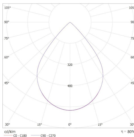
KANLUX S.A. (kat 37198) OS-M8D-WN-RX-B-P1 / Krzywa rozsyłu światła (biegunowo)
