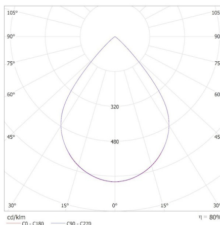
KANLUX S.A. (kat 37199) OS-H8D-WN-RX-B-P1 / Krzywa rozsyłu światła (biegunowo)
