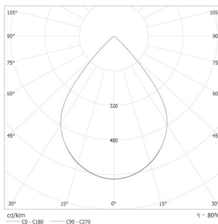
KANLUX S.A. (kat 37200) OS-S8D-NW-RX-B-P1 / Krzywa rozsyłu światła (biegunowo)
