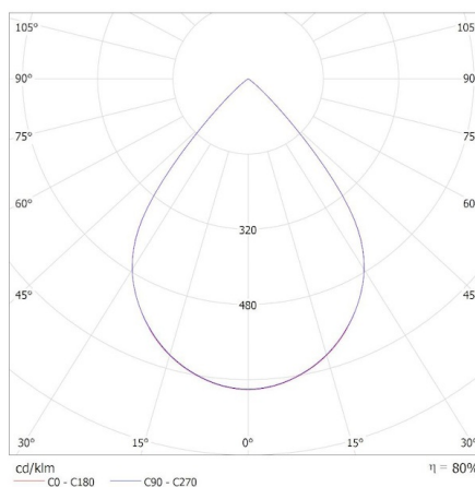
KANLUX S.A. (kat 37201) OS-L8D-NW-RX-B-P1 / Krzywa rozsyłu światła (biegunowo)
