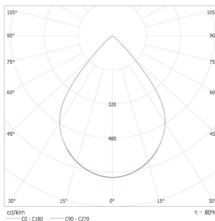
KANLUX S.A. (kat 37202) OS-M8D-NW-RX-B-P1 / Krzywa rozsyłu światła (biegunowo)
