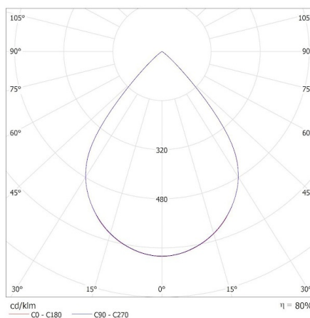
KANLUX S.A. (kat 37203) OS-H8D-NW-RX-B-P1 / Krzywa rozsyłu światła (biegunowo)
