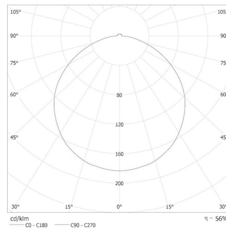
KANLUX S.A. (kat 37319) NIFU LED17,8W NW W_B / Krzywa rozsyłu światła (biegunowo)
