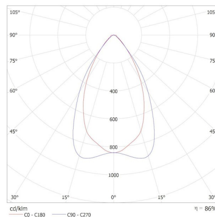
KANLUX S.A. (kat 37546) KNU-L6D-NW-B-P1D / Krzywa rozsyłu światła (biegunowo)
